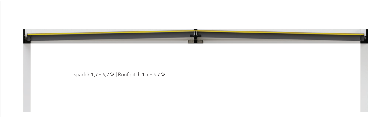
Przekrój - konstrukcja z krokiewiami (poliwęglan/szkło) | Cross-section - structure with rafters (polycarbonate/glass)
